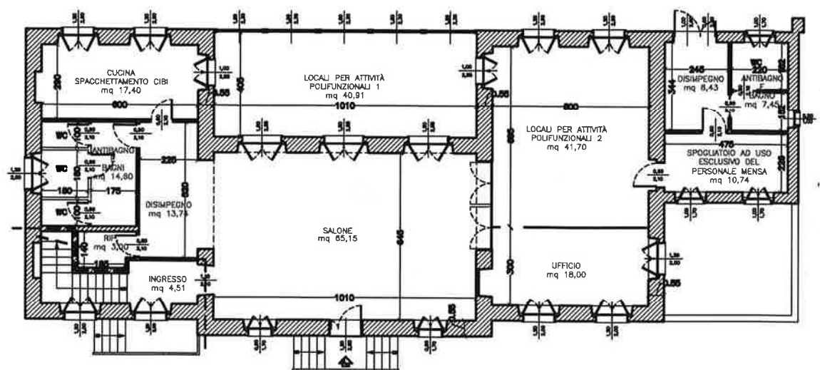
PIANTA PIANO TERRA C.A.G. CORGENO
